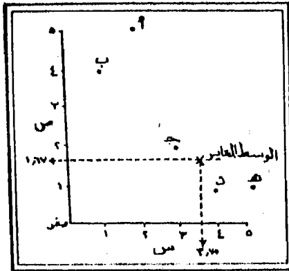
شكل (٢) الوسط الجغرافى المعايير
